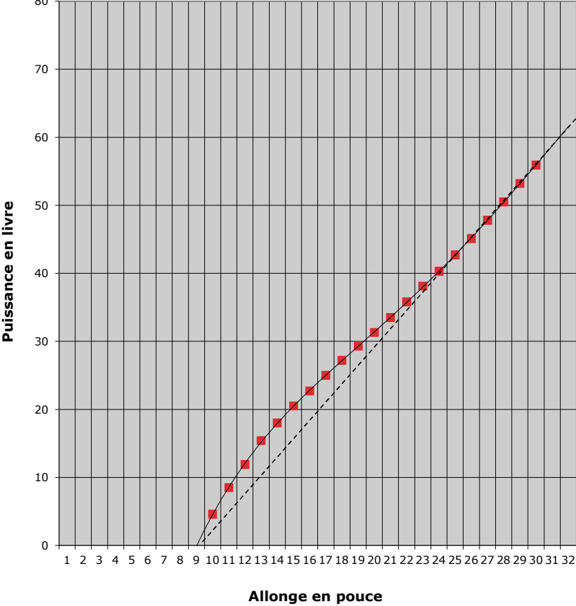
Courbe de Puissance "Phœnix Hunter 50,50"
